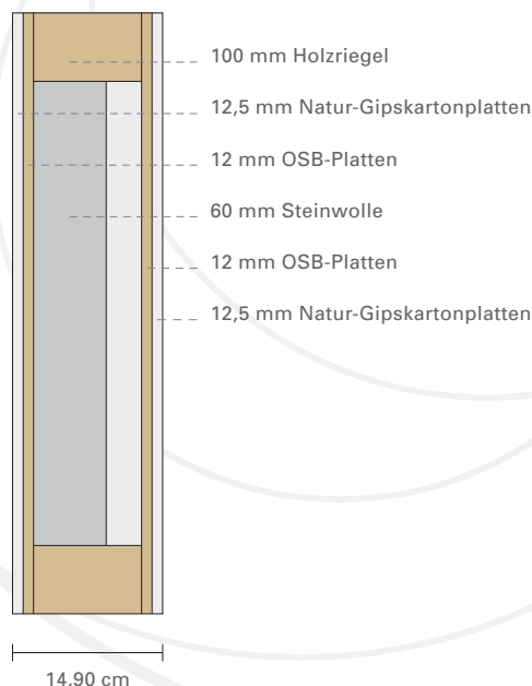
INNENWAND
