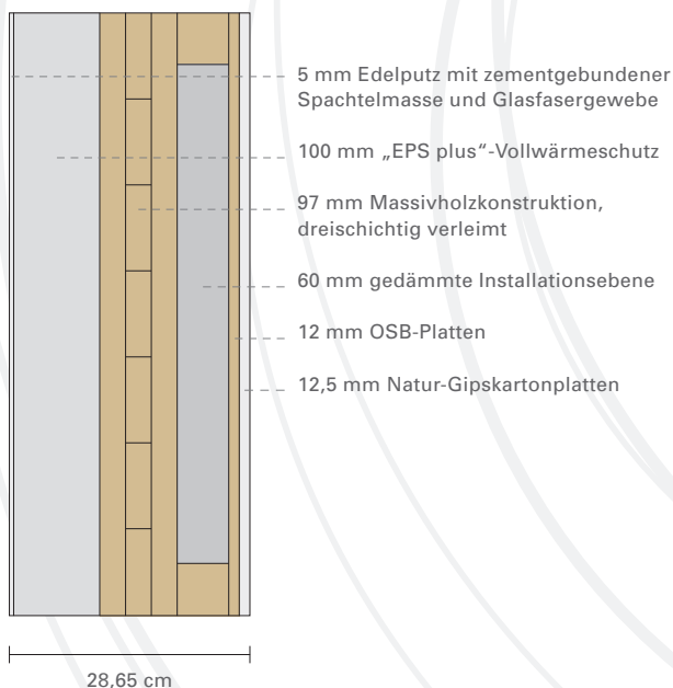
AUSSENWAND (U-WERT: 0,176 W/m 2 K)
